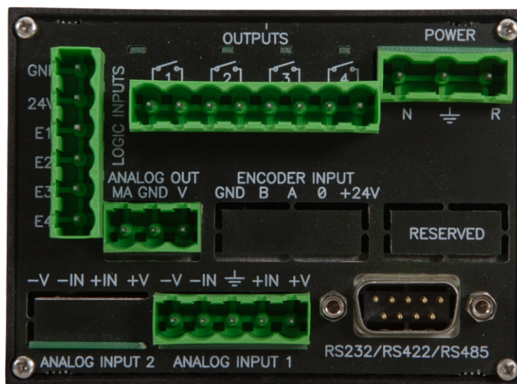
DW-M2D Vue arrière
